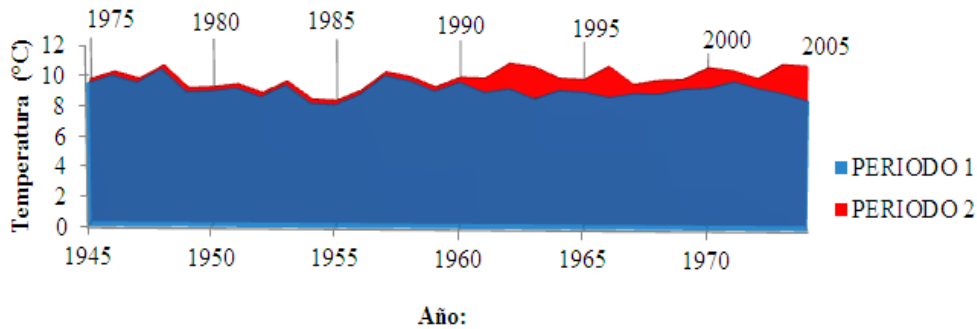
Figura 6. Incremento de las temperaturas mínimas en el periodo dos respecto al uno según la interacción periodos*años.
