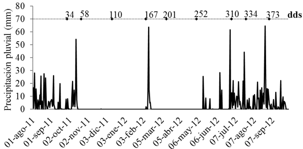
Figura 14 (13). Variaciones de lluvia durante el ciclo de plantilla del experimento de sequía realizado en el área de Tamazula, Jalisco en 2011-12 (Fuente: Lomelí-Sandoval, 2014)
