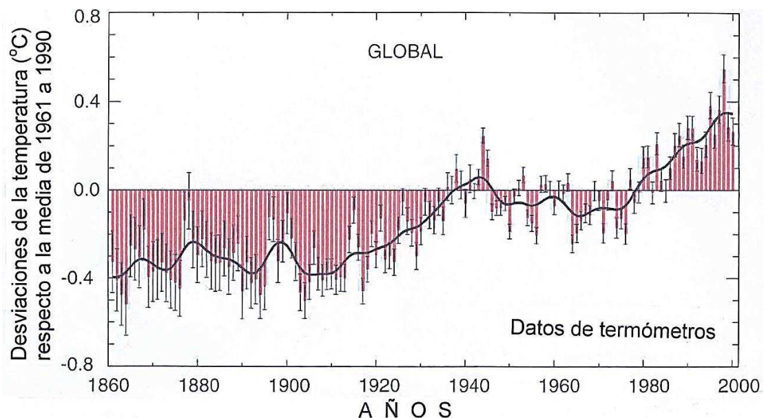
Figura 2. Desviaciones de las temperaturas (°C) de la superficie del suelo y del mar combinadas, del periodo 1861-2000 respecto al promedio del intervalo 1961-1990. Adaptación del autor en base a IPCC (2001, p 26) y con su anuencia.
