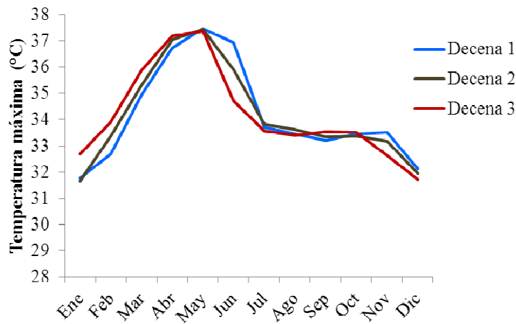
Figura 5. Variación de las temperaturas máximas de las máximas decenales en la interacción mese*decenas. Decena 1: día 1 a 10; decena 2: día 11 a 20; decena 3: día 21 a día último del mes.
