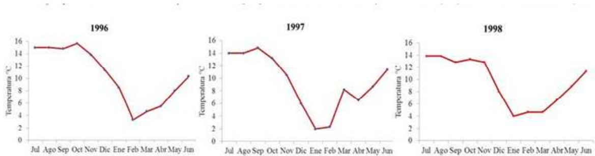
Figura 8. Se muestra la distribución de las temperaturas mínimas de las mínimas mensuales durante la GSI, en 1996 con un descenso pico en febrero, en 1997 con dos similares uno en enero y otro en febrero y en 1998 con tres similares uno en enero otro en febrero y otro en marzo.
