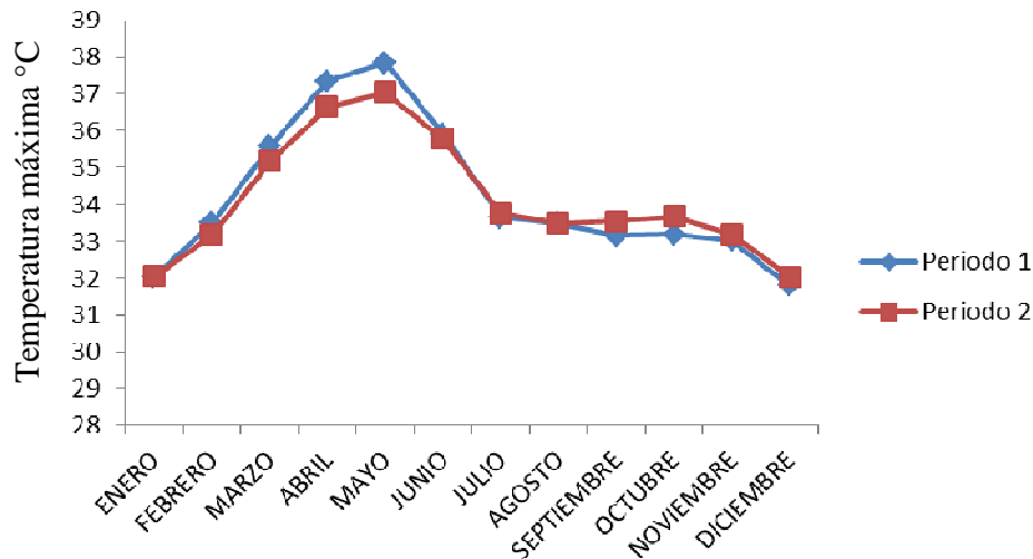
Figura 4. Variación de la temperatura máxima en la interacción periodos*meses. Periodo 1, antes de 1975 y 2, después de 1975.
