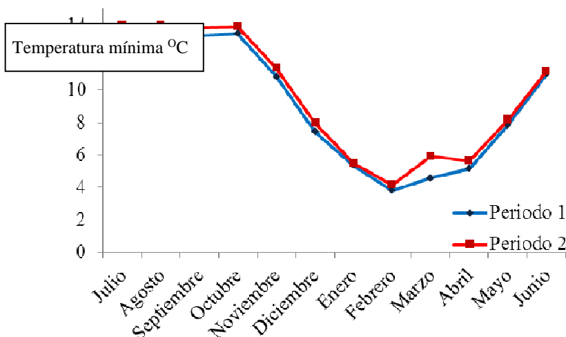
Figura 7) Variación de las temperaturas mínimas en la interacción periodos*meses con énfasis en la GSI.
