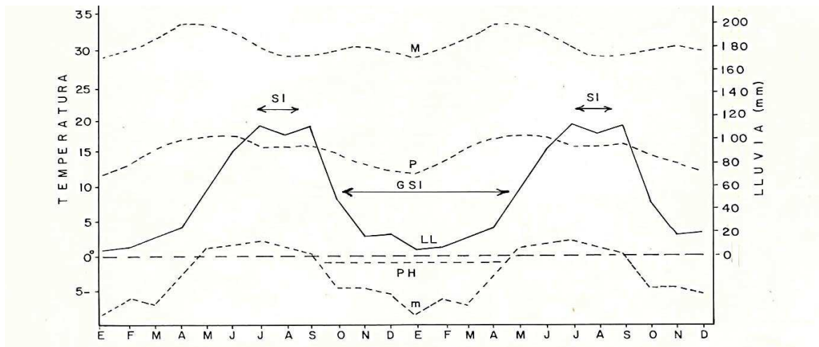
Figura 1. Distribución de las temperaturas (°C) máximas (M), lluvia mensual (LL), temperaturas mínimas (m); al unir dos años se aprecia la Gran Sequía Invernal (GSI), el periodo de heladas (PH) y el descenso de lluvia que ocurre en esta localidad en agosto o Sequía Intraestival (SI), en Teotihuacán, Estado de México, 19°40'54.94" N, 98°51'59.77" O, elevación 2277 m.
