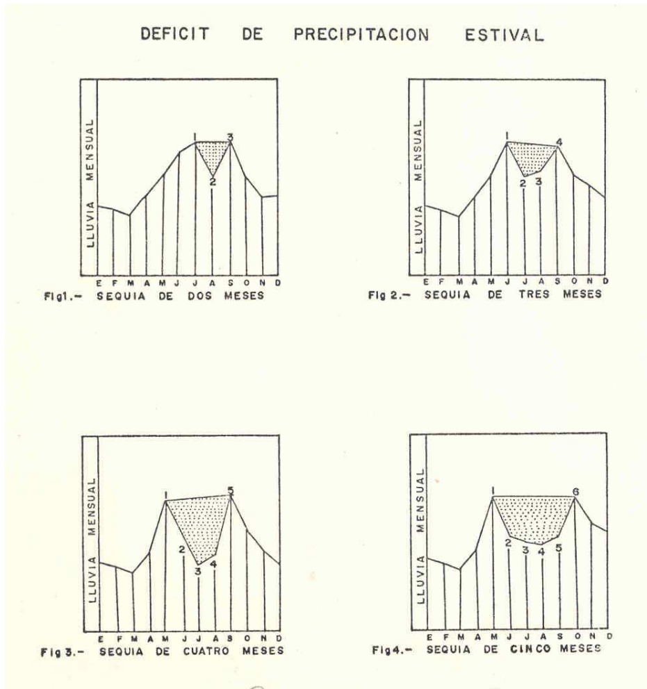
Figura 3. déficits de la Sequía Intraestival (SI): Fig 1 cuando es de dos meses; Fig 2 cuando es de tres meses; Fig 3 cuando es de cuatro meses; Fig 4 cuando es de cinco meses. Adaptación de los autores en base a la fuente: Reyna, (1970).
