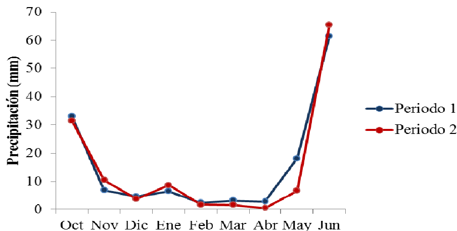
Figura 9 (3. 1) Interacción periodos*meses en relación a la precipitación decenal en el lapso en que ocurre la GSI.
