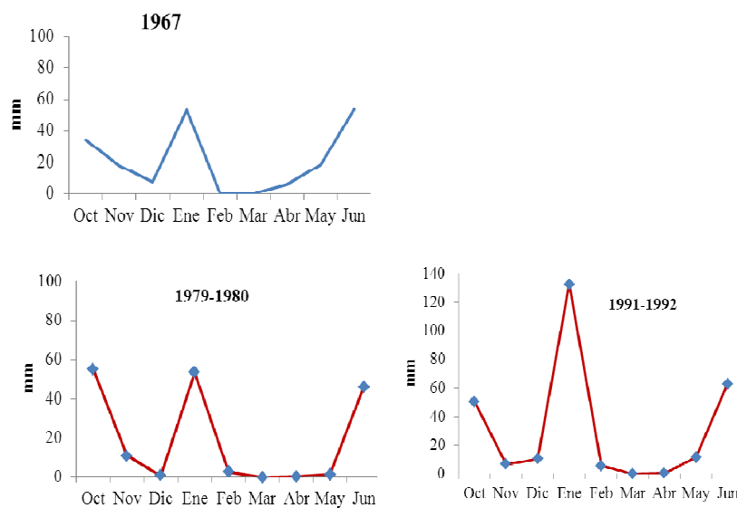
Figura 13 (14). Variaciones de lluvia dentro de la GSI, ocurridas específicamente en el mes de enero.
