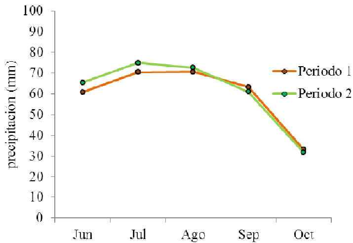
Figura 11. Efecto de la interacción meses*periodos sobre la lluvia, en el lapso en que suele ocurrir la SI.
