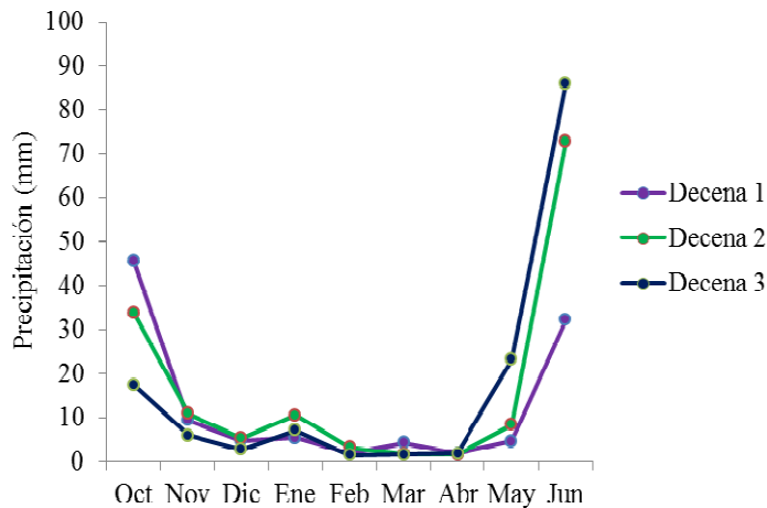
Figura 10 (3. 2) Interacción meses*decenas en relación a la precipitación en el lapso en que ocurre la GSI
