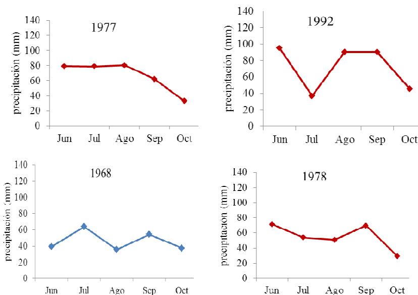
Figura 12. Muestra las principales variaciones de la SI: ausente en 1977, presente en julio de 1992, en agosto de 1968 y con duración de dos meses en julio y agosto de 1978. Fuente: Lomelí-Sandoval, 2014)
