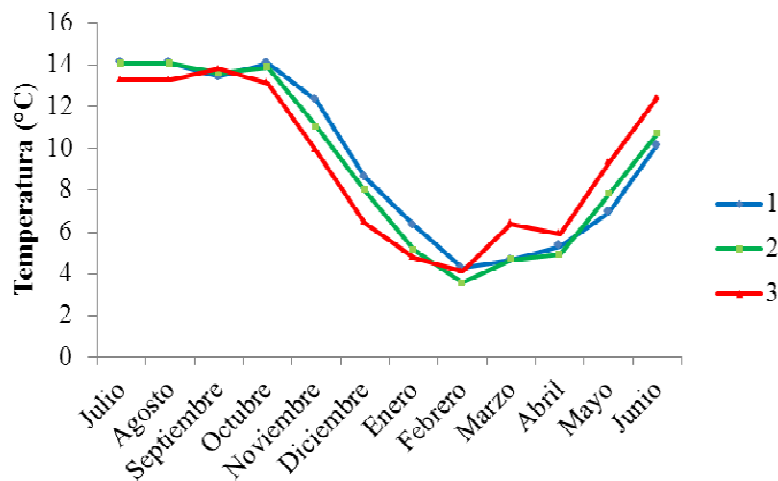
Figura 8. Variación de la temperatura mínima en la interacción meses*decenas con énfasis en la GSI.
