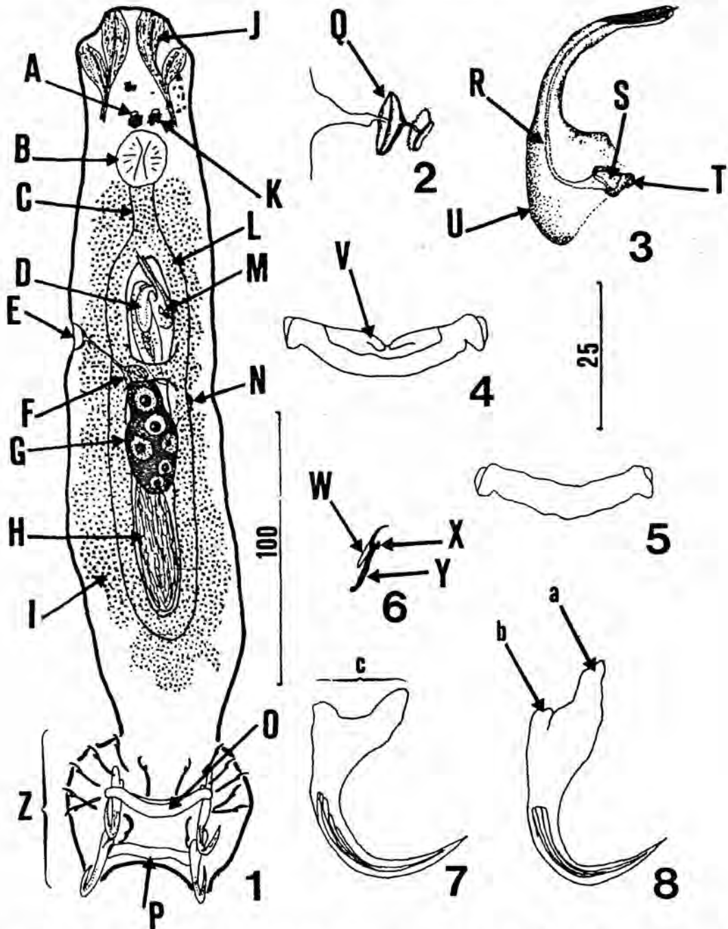
Figura 1. Sciadiclithrum mexicanum . 1. Gusano completo en posición ventral. 2. Vagina. 3. Complejo copulador. 4. Barra ventral. 5. Barra dorsal. 6. Microgancho. 7. Macrogancho ventral; c. Base del macrogancho ventral. 8. Macrogancho dorsal; a. Raíz superficial; b. Raíz profunda. A. Lente conspicuo. B. Faringe. C. Esófago. D. Reservorio prostático. E. Abertura vaginal. F. Receptáculo seminal. G. Ovario. H. Testículo. I. Vitelógenas. J. Glándulas cefálicas. K. Ocelos. L. Intestino. M. Órgano copulador masculino (MCO). N. Vas deferens. O. Barra ventral. P. Barra dorsal. Q. Esclerita vaginal. R. MCO. S. Base del MCO. T. Elongación de la base del MCO. U. Pieza accesoria. V. Cavidades membranosas. W. Filamento (domus). X. Pulgar (thumb). Y. Pie (shank). Z. Haptor. Todas las figuras corresponden a la escala de 25 \mu\text{m} , excepto para la figura 1 (100 \mu\text{m} ) (modificado de Kritsky, Vidal-Martínez y Rodríguez-Canul, 1994).
